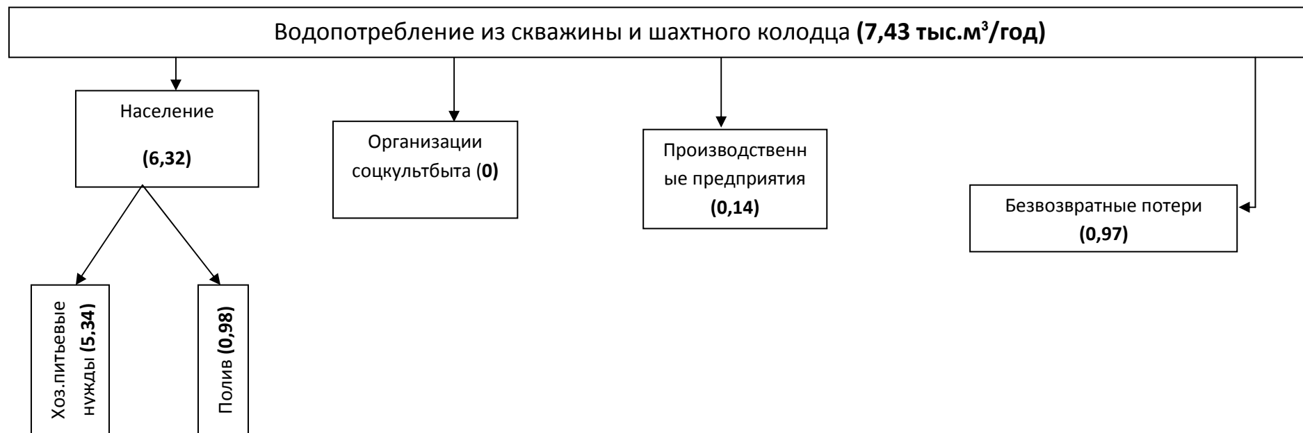
Балансовая схема водопотребления а. Тумба (тыс.м 3 /год)
